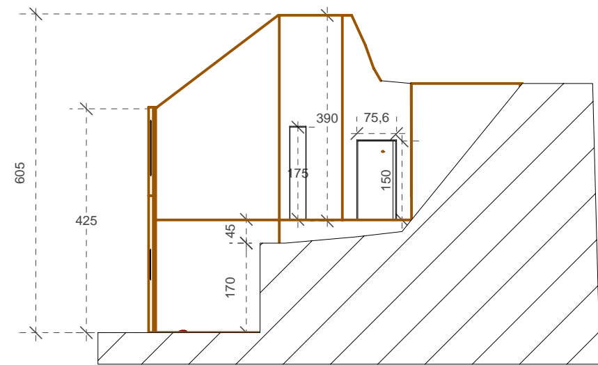
FACADE EST
